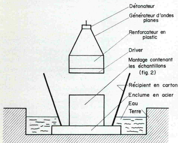
FIG. 1. Dispositif expérimental de choc.
